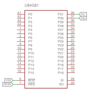
P8X32A-M44
