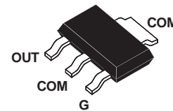
SOT-223 ACS108-5SN
